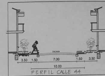
PERFILES VIALES
